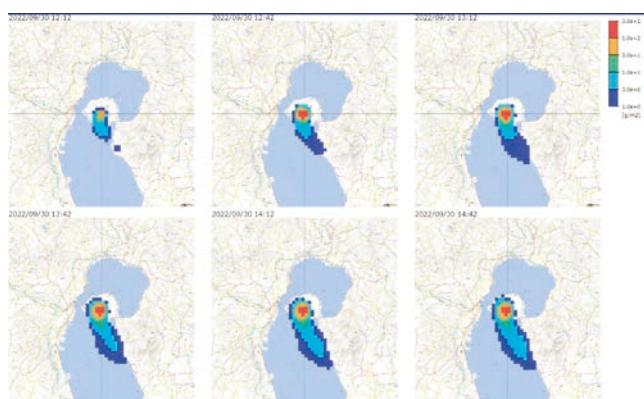
図2 2022年9月30日の桜島噴火後の降灰量の予測。連続化シミュレータにより火山灰噴出率に基づいて6分ごとに降灰量を予測することができます。
