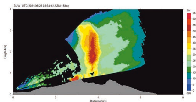
図1 レーダーで捉えた2021年8月28日の諏訪之瀬島噴火の噴煙。火口上3km以上の高さまで達しています（噴煙濃淡を色で表現）。
