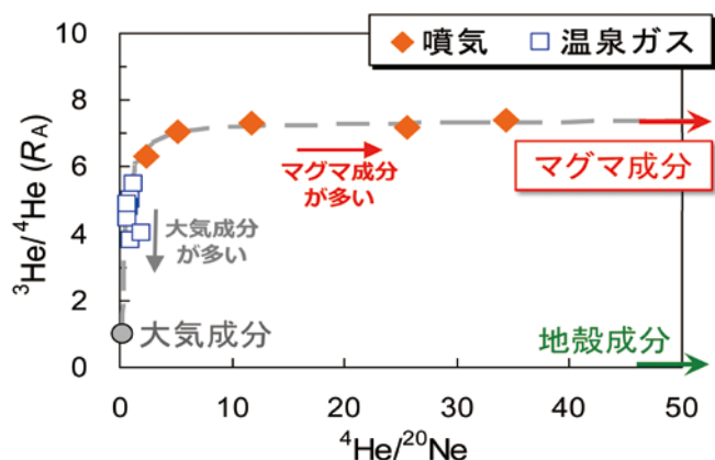
図1 草津白根山の噴気と温泉ガスの ^3\text{He}/^4\text{He} 比と ^4\text{He}/^{20}\text{Ne} 比。
