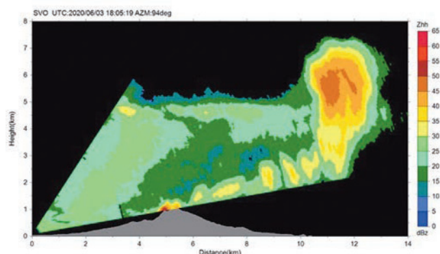
図1 レーダーで捉えた2020年6月4日の桜島噴火の噴煙。火口上7km以上の高さまで達しています（噴煙濃淡を色で表現）。
