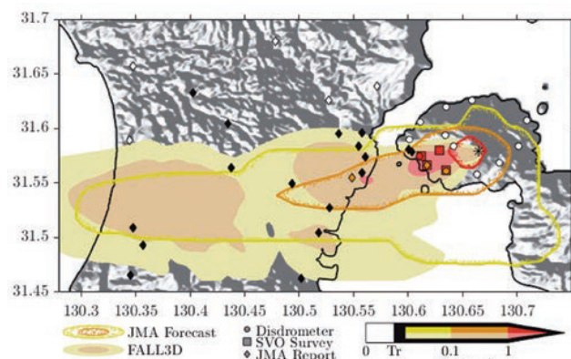
図2 2018年6月16日の桜島噴火後の降灰量の予測。高解像度の風と正確な噴出速度により、予測を改善することができます。
