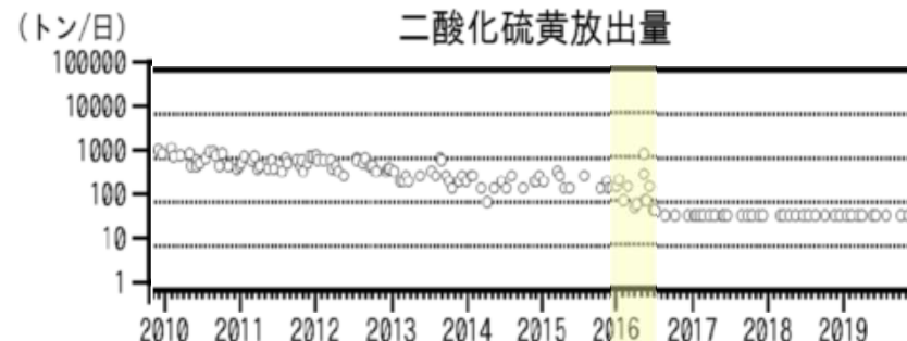
三宅島の長期的な活動推移 (第145回火山噴火予知連絡会 気象庁資料)
