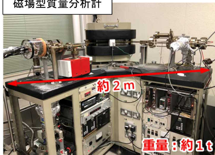
磁場型質量分析計
