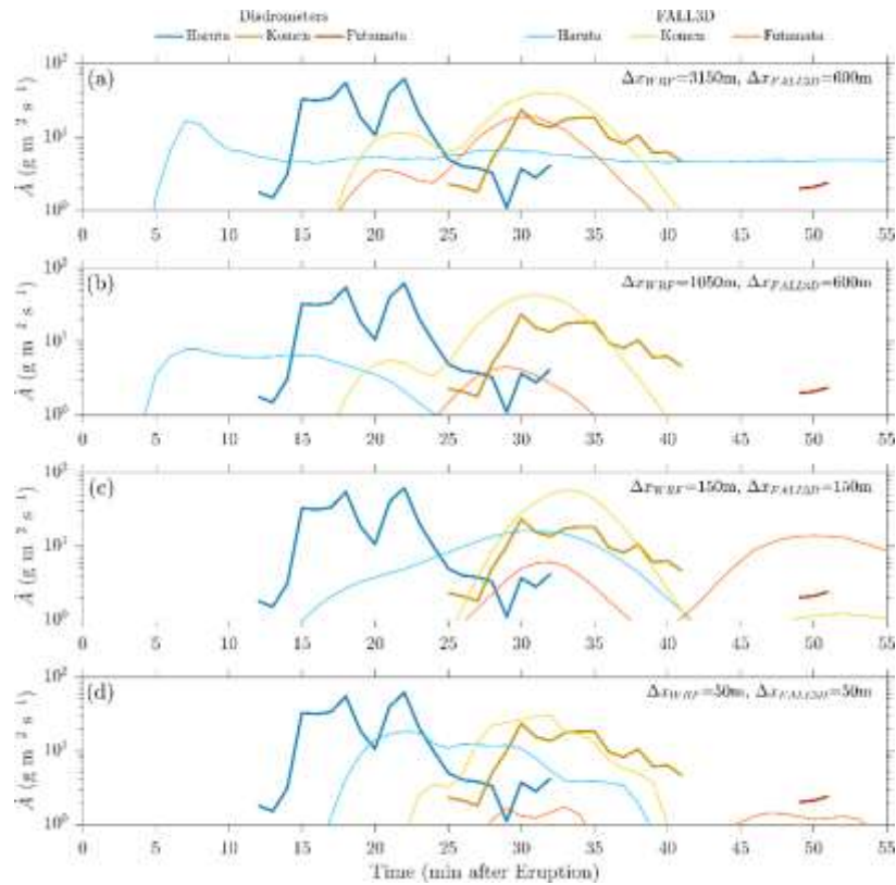
図 90 ハルタ山（青）、高免（黄）、二股（赤）における降灰量の時系列。太い実線はディスドロメータによる観測値、細い実線は計算値を示す。計算値は、異なる解像度の結果をパネル毎に示す。
