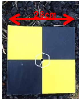
図 5 対空標識
