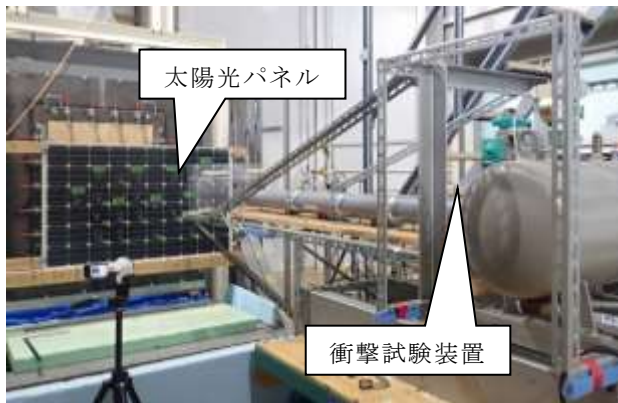
(左) 太陽光パネルの噴石に対する耐衝撃性能試験の実験装置。(右) 衝撃後の円状にひび割れた（カバーガラスが割れた）状態。
