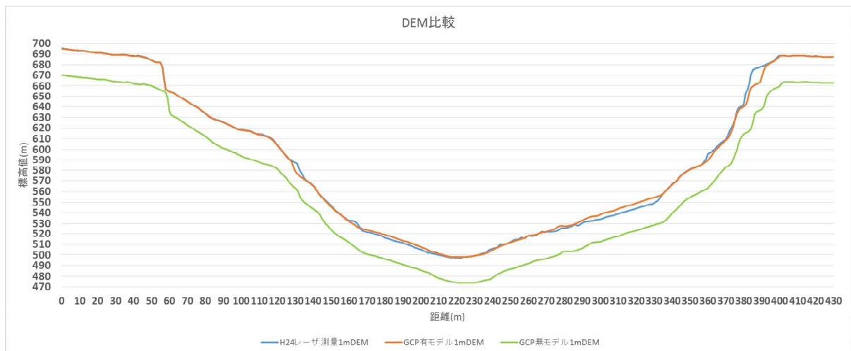
図 13 H24レーザ測量データ・GCP有モデル・GCP無モデルの1mDEM比較結果
