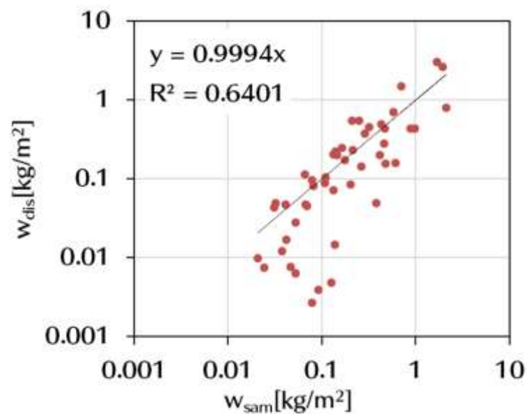
図 52 採取された火山灰重量から求めた降灰量と、同時時間帯に観測されたディストロメータの観測値から経験的な式により計算された降灰量の相関。
