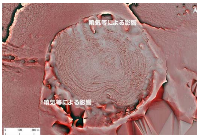
図 6 噴火後の新燃岳火口周辺の 3 D モデル (2018 年 3 月 9 日 15 時頃)
